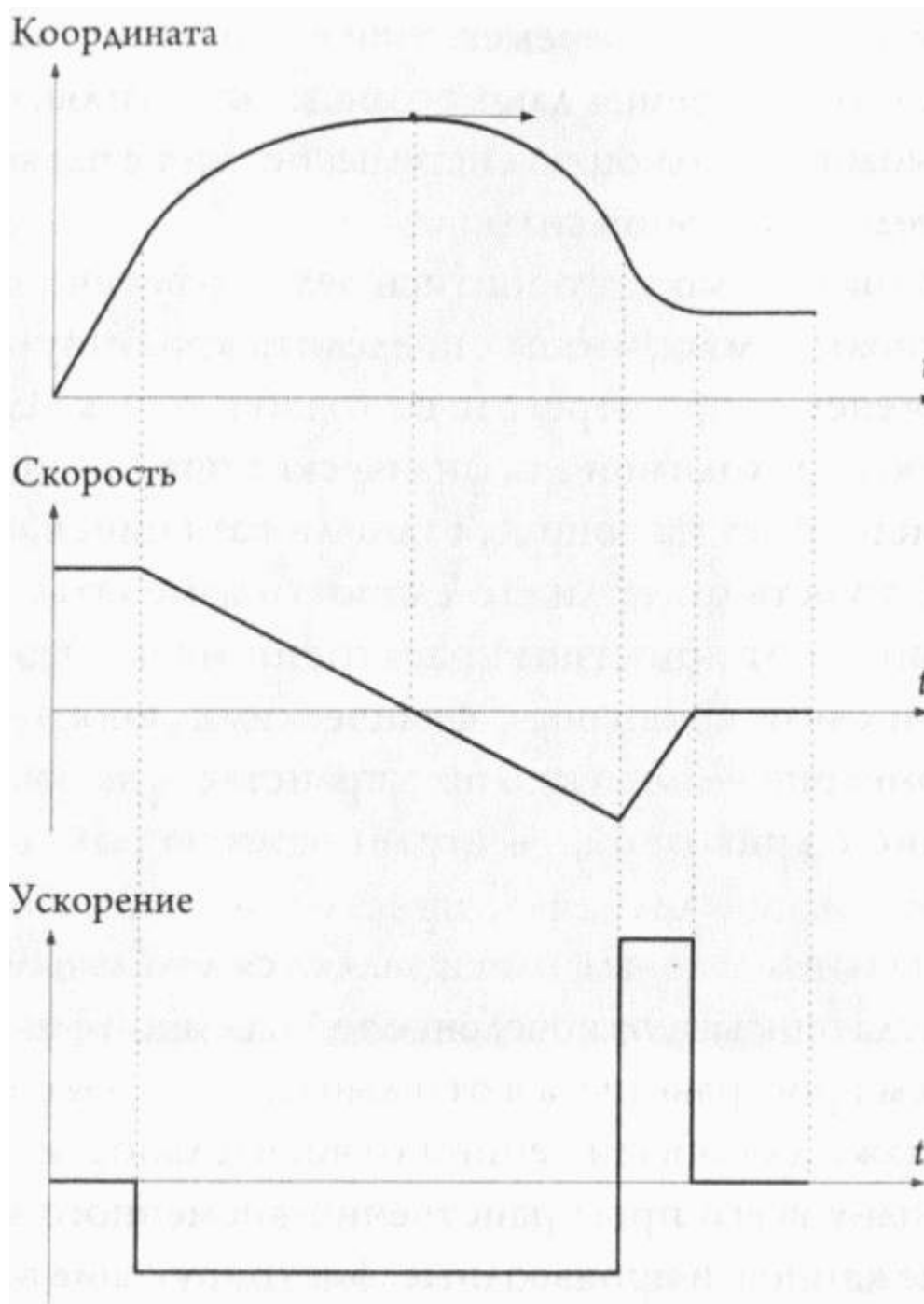
Рис. 3.2. Графики, иллюстрирующие движение объекта вдоль определенной траектории. Скорость – величина, показывающая, насколько быстро положение объекта изменяется с течением времени, может быть получена путем взятия производной по кривой перемещения. Производная определяется наклоном кривой в данной точке и численно равна скорости в соответствующий момент времени. Ускорение, величина которого показывает, как изменяется скорость с течением времени, можно, в свою очередь, получить, взяв производную по кривой зависимости скорости от времени. Значение ускорения в определенный момент времени определяется наклоном кривой в соответствующей точке
