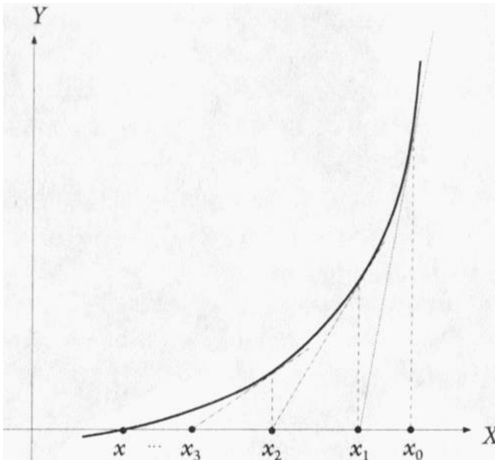
Рис. 5.2. Наглядная иллюстрация метода Ньютона. Для того чтобы найти точку пересечения определенной кривой или функции с осью X , сначала нужно наугад подобрать некую точку x_0 наиболее подходящую для этого. Затем необходимо провести касательную к кривой в точке x_0 и отметить точку, в которой эта касательная пересечет ось X (это будет точка x_1 ). В том случае, если наше изначальное предположение не было полностью ошибочным, продолжая этот процесс, мы будем получать точки все ближе и ближе к искомой
